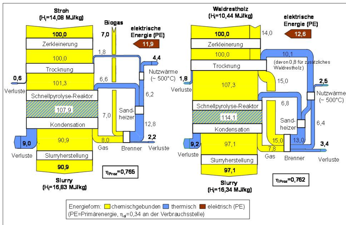
Abb. 2: Energiebilanzen zur Schnellpyrolyse von Stroh und Waldrestholz
